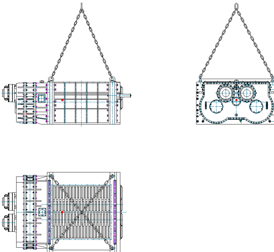
图 4-1 如何起吊破碎机
