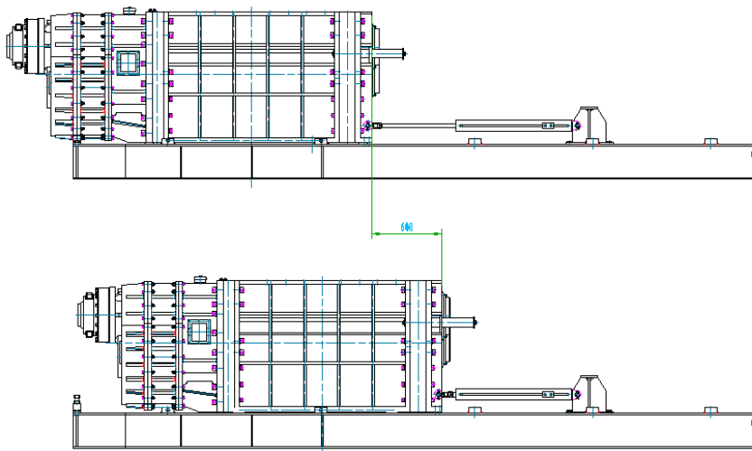
图 6-1 破碎机检修移动示意图
