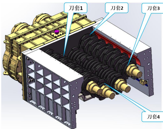
图 6-4 刀盘的拆卸状态
